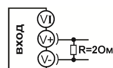
Токовый вход 0...40 \text{ мА}
