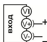
Потенциальный вход -10...80 \text{ мВ}
